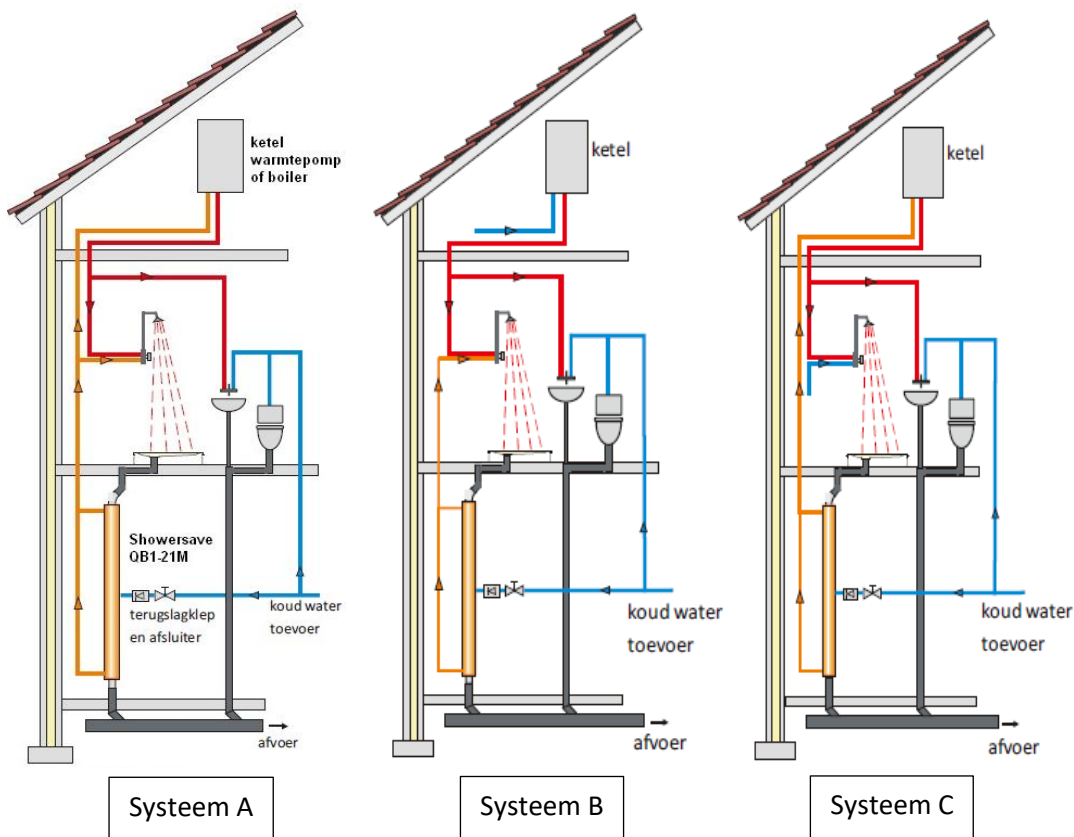
Aansluitschema's Showersave®QB1-21M
