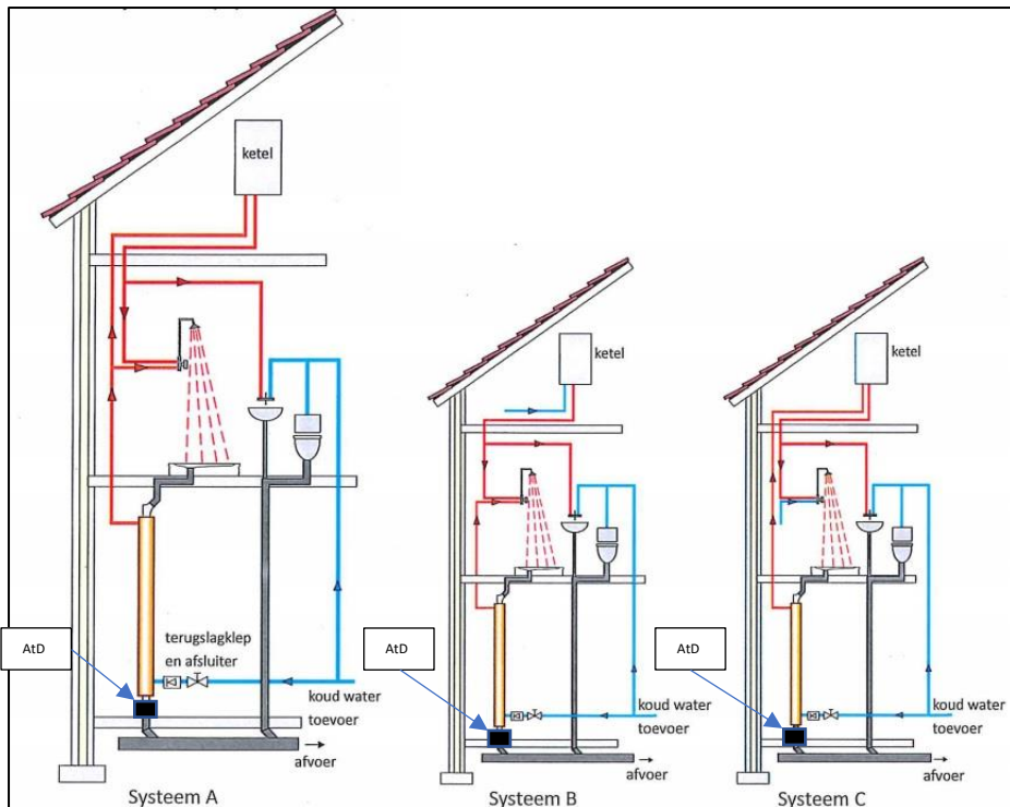
Aansluitschema's ShowerSave®QB2-21
